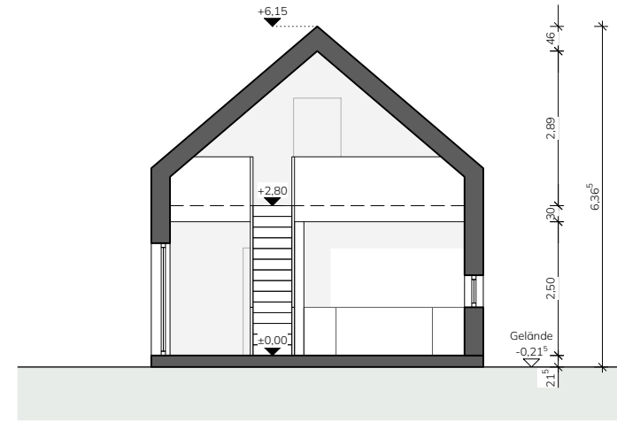
SCHNITT
