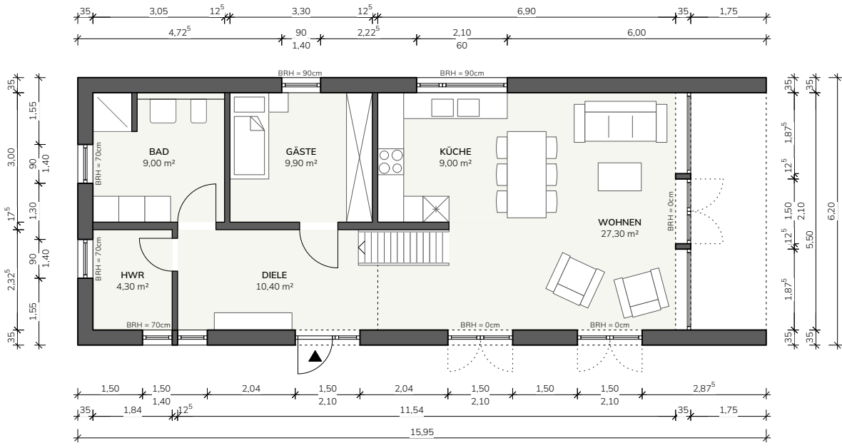
ERDGESCHOSS
