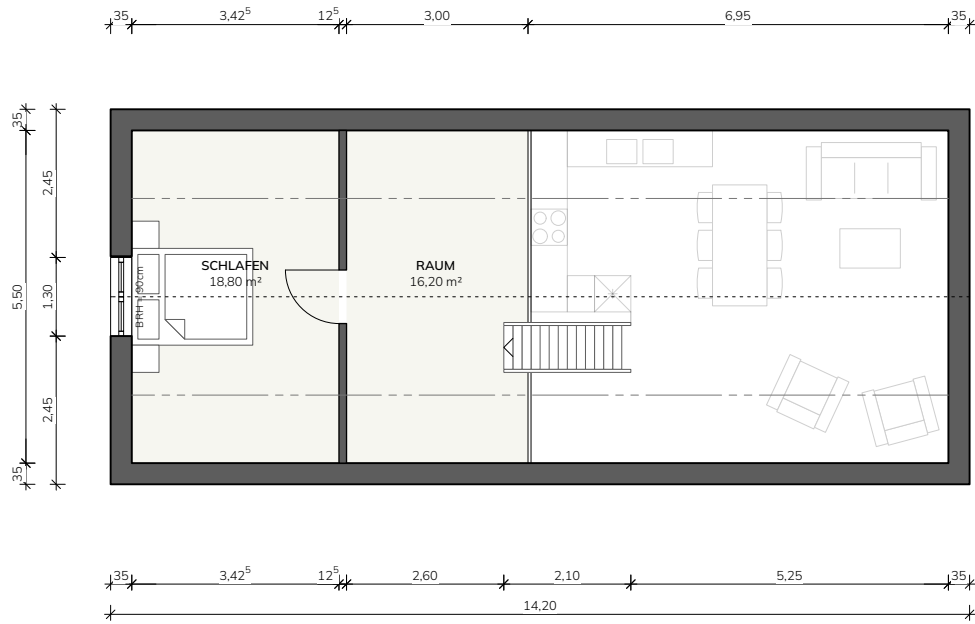
OBERGESCHOSS
