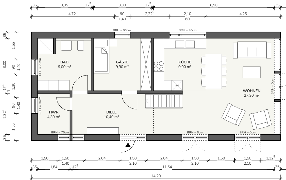
ERDGESCHOSS
