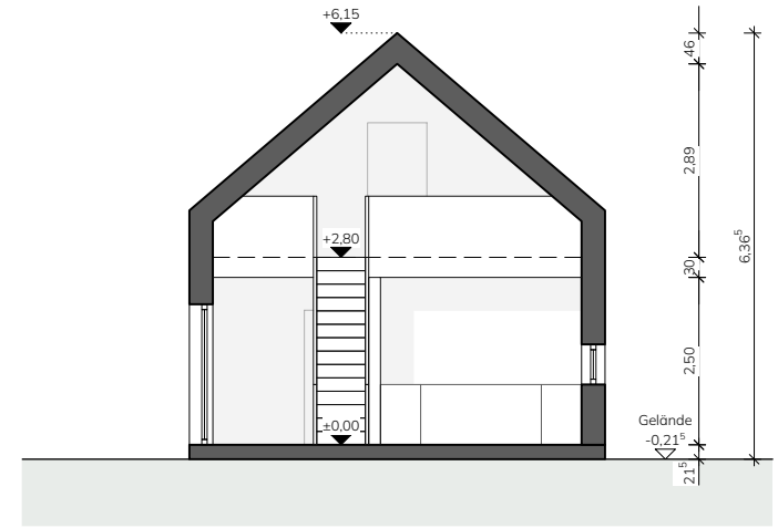
SCHNITT
