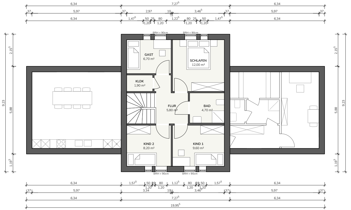
GRUNDRISS OG
