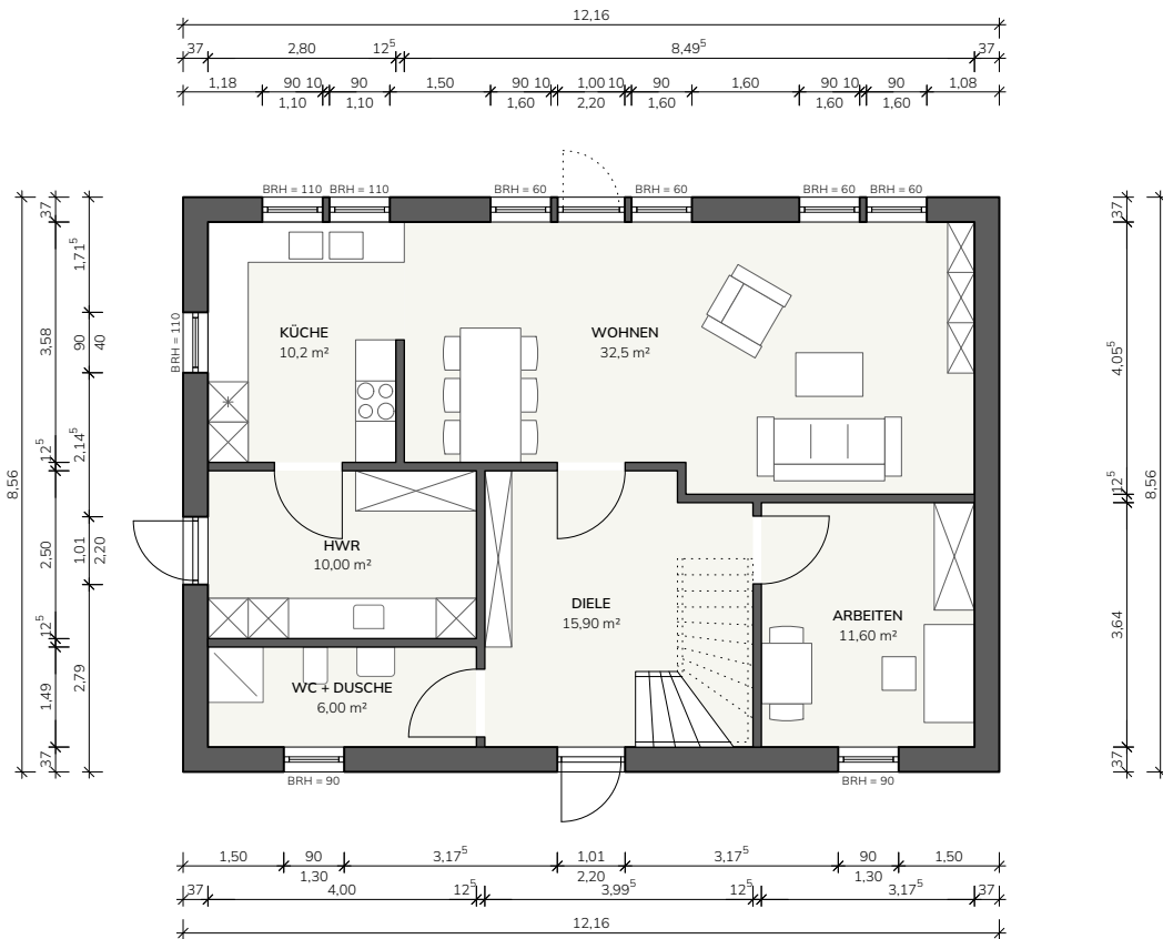
GRUNDRISS EG
