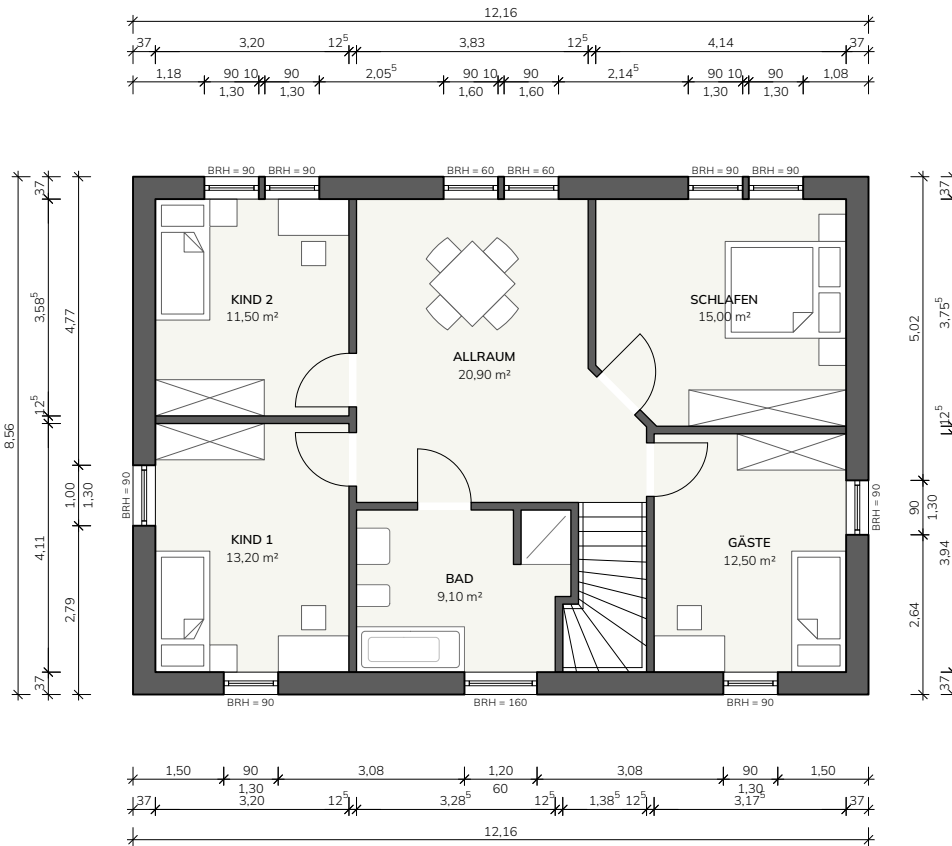
GRUNDRISS OG
