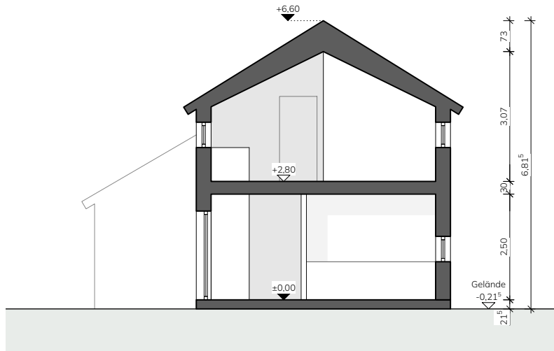
SCHNITT
