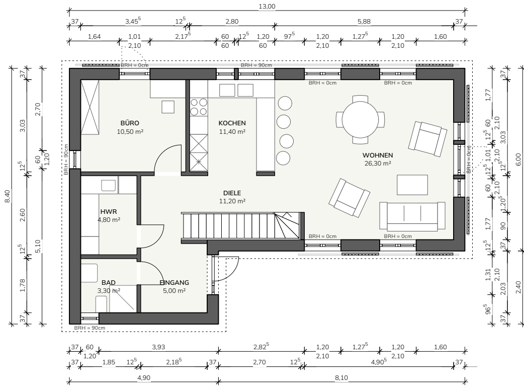
ERDGESCHOSS
