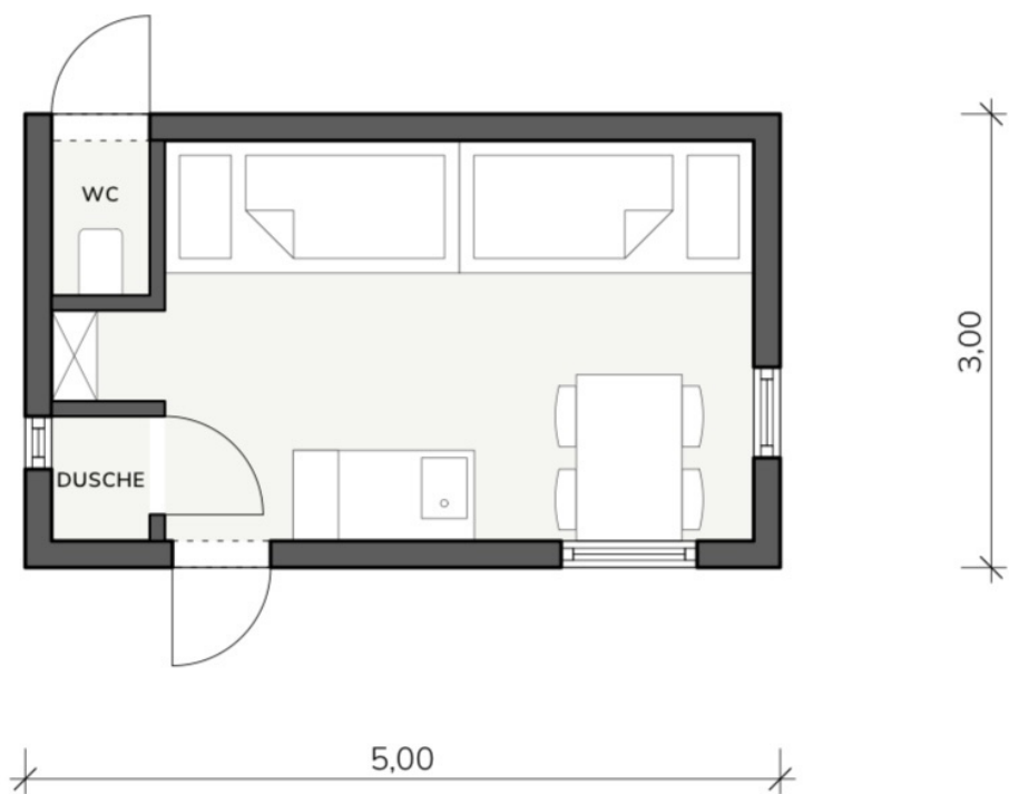
GRUNDRISS - VAR.1
