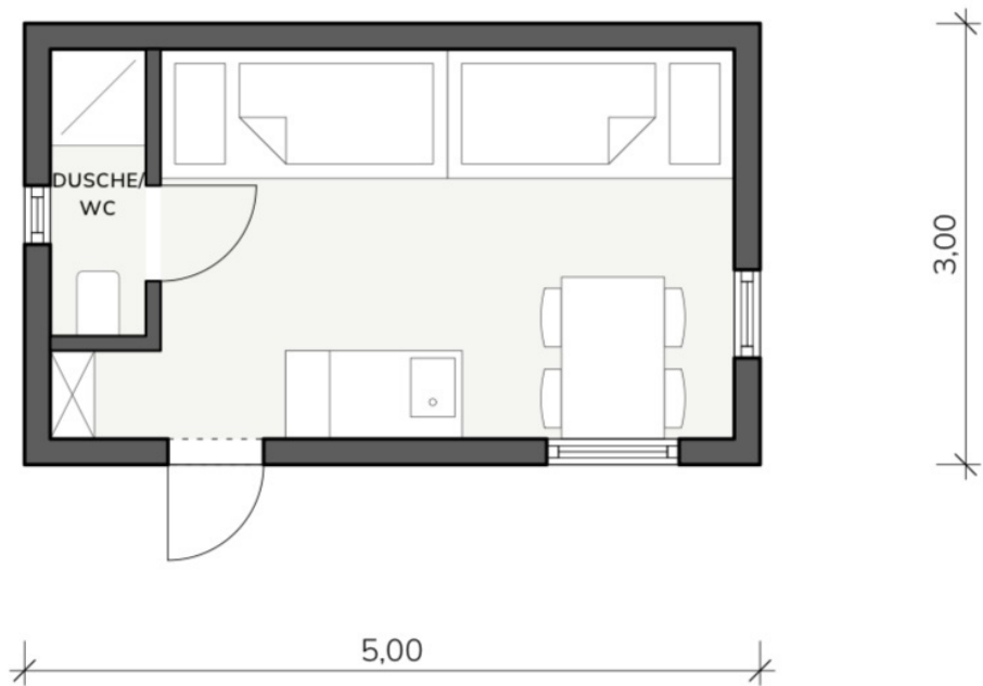
GRUNDRISS - VAR.2
