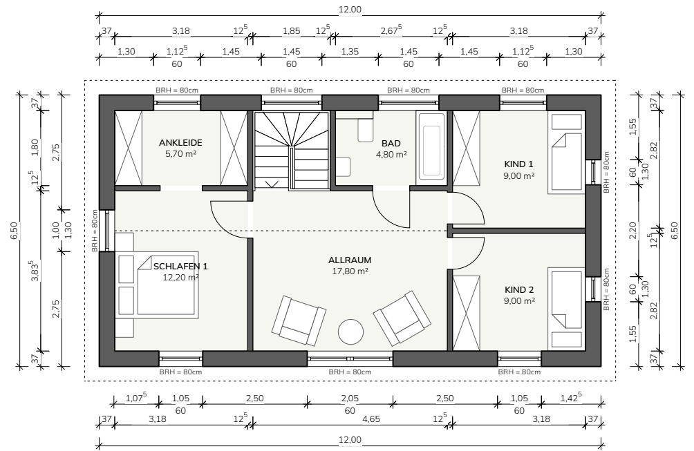
OBERGESCHOSS
