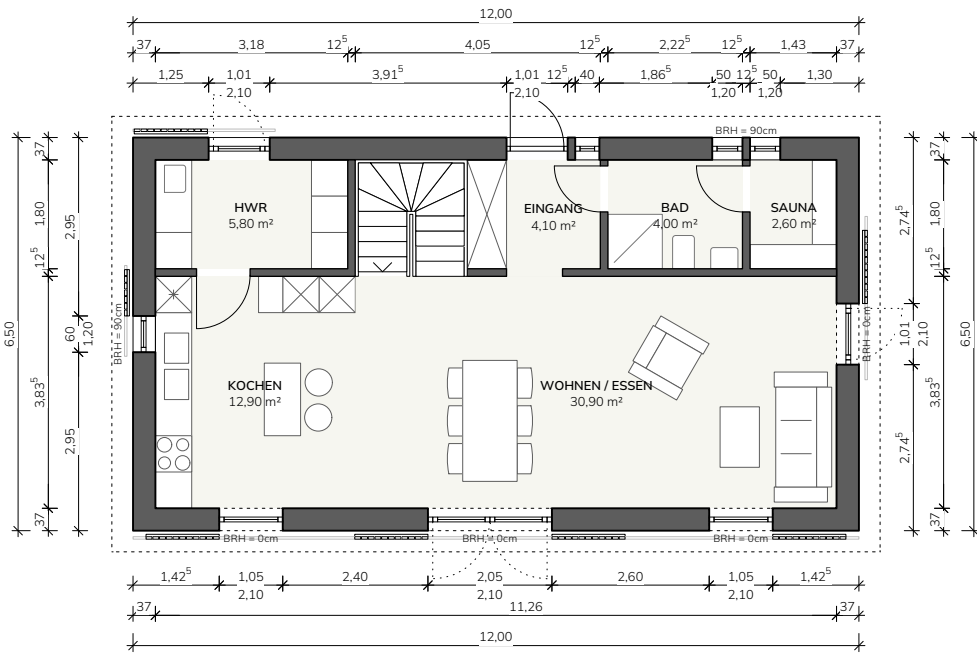
ERDGESCHOSS
