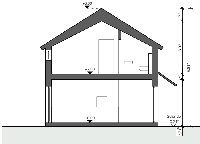
SCHNITT
